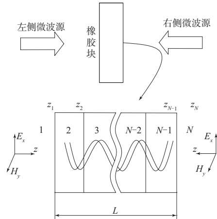
图2 多层橡胶复合材料微波加热物理模型
