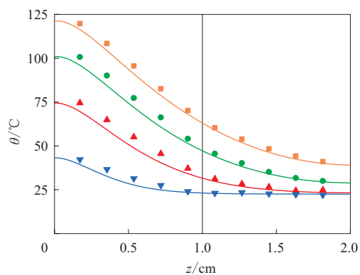
图9 单波源下两层橡胶复合材料的温度分布曲线 (上SBR材料下NBR材料)
